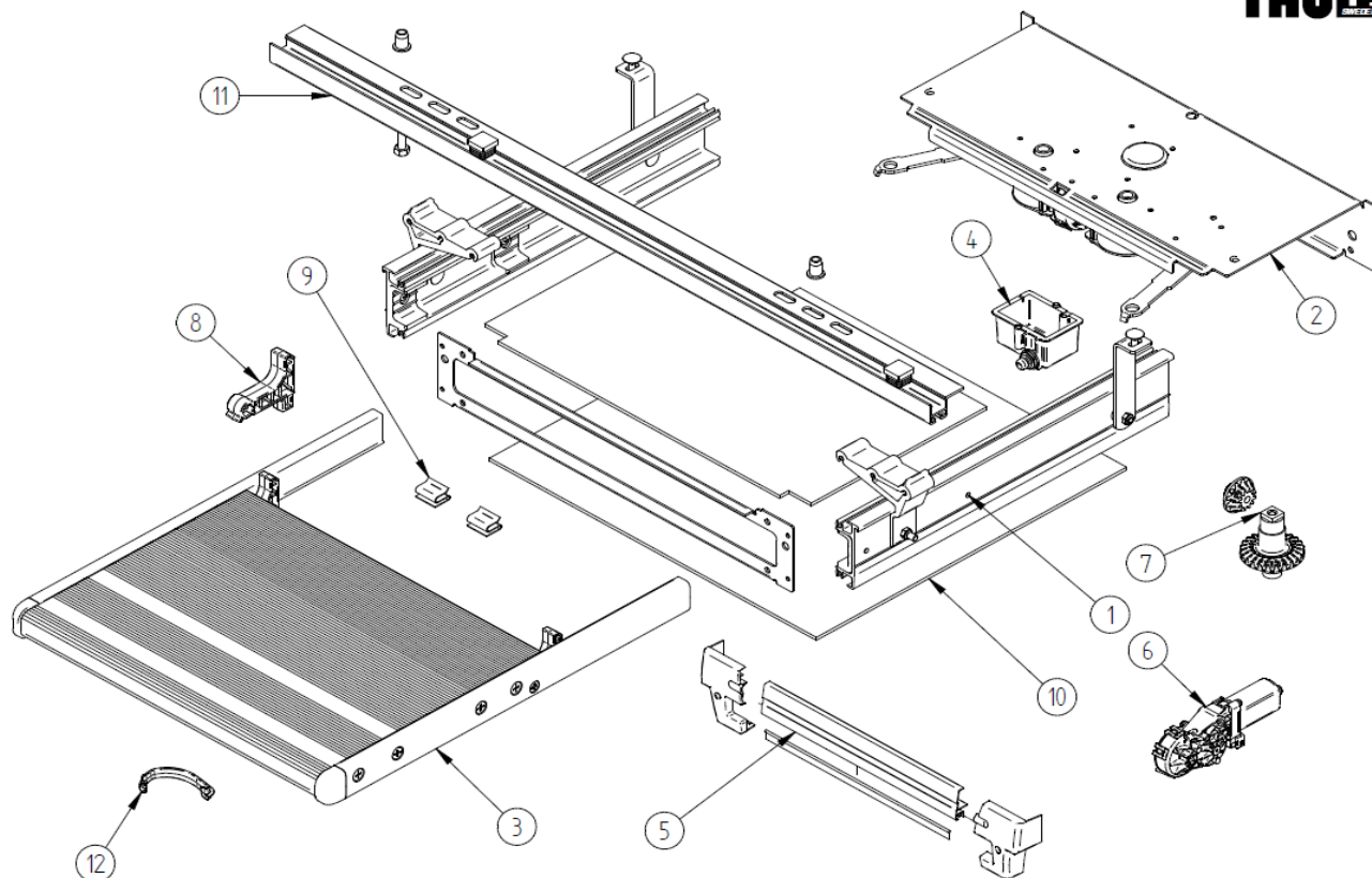
THULE Slide out Ducato V16
